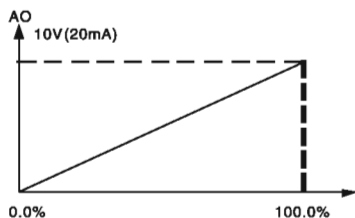
图6-13 给定量与模拟输出对应关系
