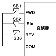
图 6-11 三线式控制模式 2
