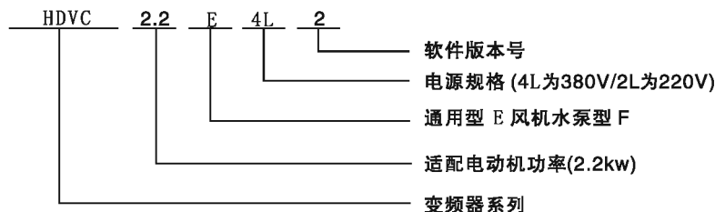
图 1-1 变频器铭牌说明
