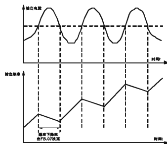
图 6-23 限流失速功能
