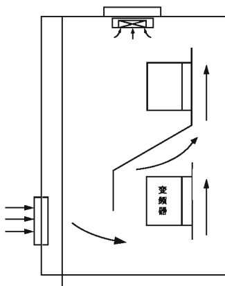
图 3-3 多台变频器的安装
