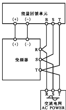
图 4-17 能量回馈单元连接图
