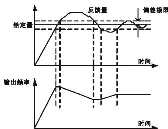
图6-19 偏差极限与输出频率的对应关系
