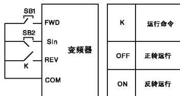
图6-10 三线式控制模式1
