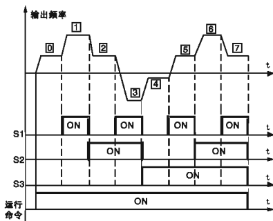
图 6-20 多段速度运行逻辑图
