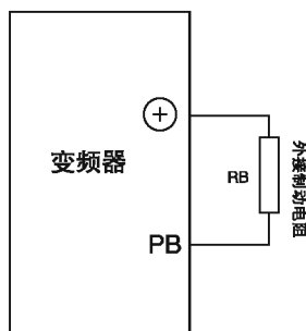
图 1-11 制动电阻的安装
