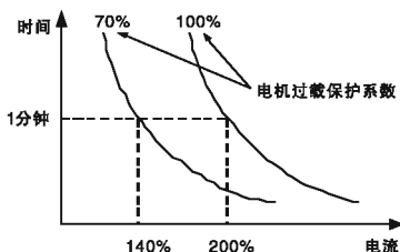
图6-21 电机过载保护系数设定
