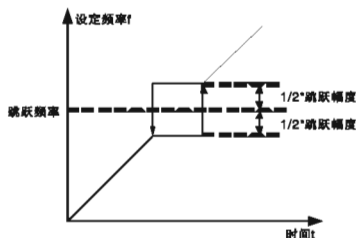
图 6-14 跳跃频率示意图
