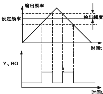
图6-17 频率到达检出幅度示意图
