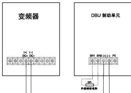
图 1-12 制动单元的连接
