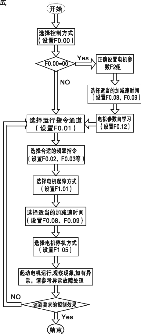
图 5-6 快速调试流程图
