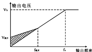
图 6-7 手动转矩提升示意图
