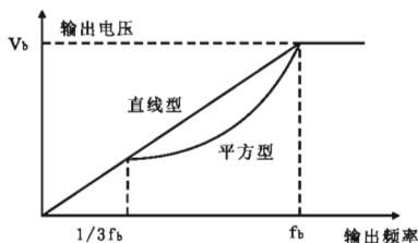
图6-6 V/ F 曲线示意图
