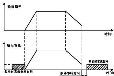
图6-3 直流制动示意图
