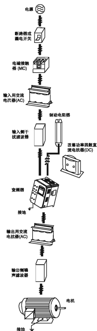
图 4-1 外围设备的连接图
