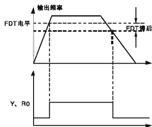
图6-16 FDT 电平示意图
