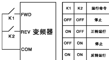
图 6-9 两线式控制（使能与方向分离）
