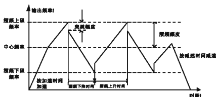
图6-15 摆频运行示意图
