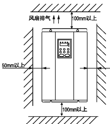
图 3-2 安装的间隔距离
