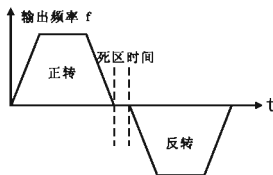
图6-4 正反转死区时间示意图
