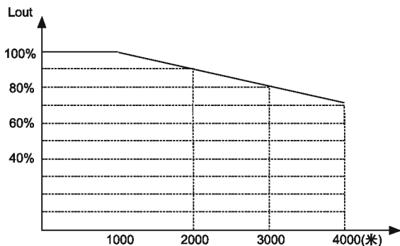
图 3-1 安装地点的海拔高度
