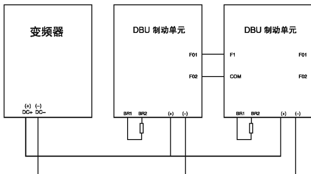
图 1-13 制动单元的并联连接
