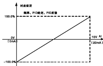
图6-12 模拟给定与设定量的对应关系
