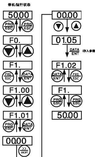
图 5-2 三级菜单操作流程
