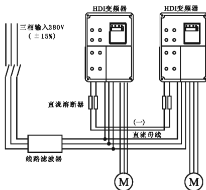
图 4-18 共直流母线的连接
