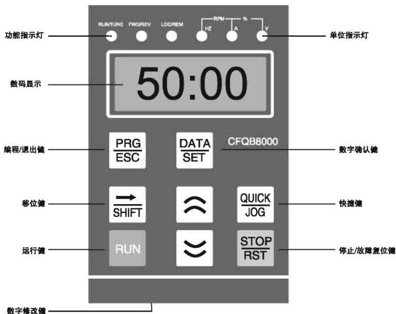
图 5-1 操作面板示意
